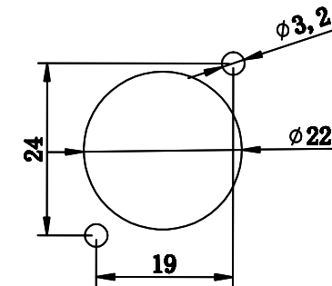
Frontplattenausschnitt (Rueckseite) Panel cut out (rear side)
