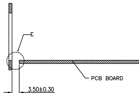
DETAIL A-A
