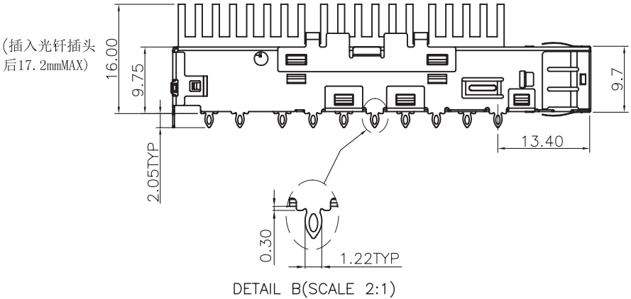
DETAIL B(SCALE 2:1)
